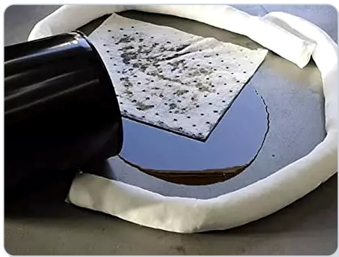
Anillo de cordón conteniendo un derrame de aceite
