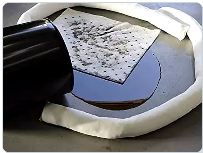
Rękaw otaczający wyciek oleju
